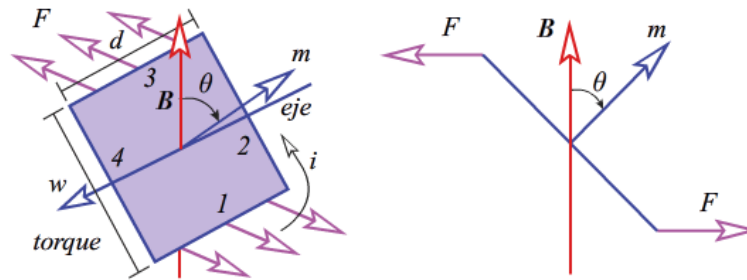
Fig.28. Se muestra una espira montada sobre un eje dentro de un campo magnético. Las fuerzas sobre las corrientes en los segmentos 1 y 3 de la espira generan una torca alrededor del eje.
