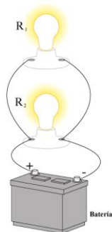
Fig. 41. Circuito con resistencias en paralelo con una batería.
