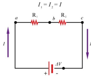
Fig. 39. Circuito mostrando el sentido de la corriente y el voltaje aplicado.
