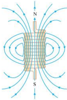
Fig. 30. Se muestran las líneas de campo de un solenoide ideal.
