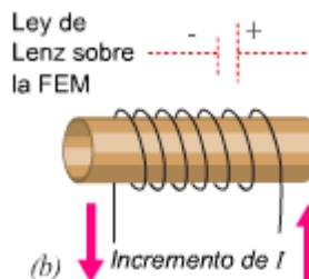
Fig. 52. La FEM autoinducida es contraria al cambio cuando la corriente aumenta.
