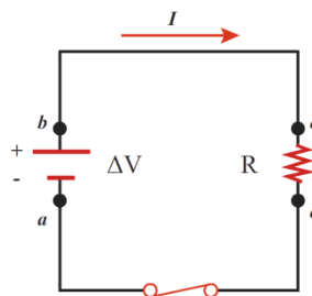
Fig.28. Circuito con una resistencia y una batería.
