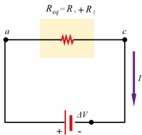
Fig. 40. Resistencia equivalente de dos resistencias en serie.
