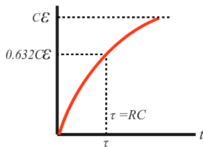
Fig. 48. Carga del condensador.
