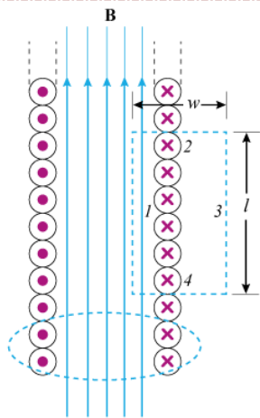
Fig. 31. Trayectoria que se evalúa para calcular el campo magnético de un solenoide ideal.
