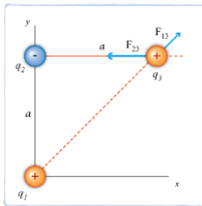
Fig. 8. Se muestra la fuerza que se ejerce sobre una partícula cargada positivamente debido a dos partículas cargadas.
