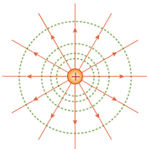
Fig.20. Líneas de campo eléctrico y las superficies equipotenciales mostradas con líneas punteadas.
