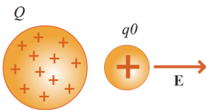
Fig. 9. Carga de prueba en el campo eléctrico de una distribución de cargas.
