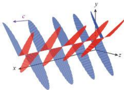
Fig. 34. Onda electromagnética.
