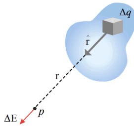
Fig. 14. Elemento infinitesimal de carga \Delta q a una distancia r del punto.
