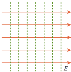
Fig. 19. Superficies equipotenciales.
