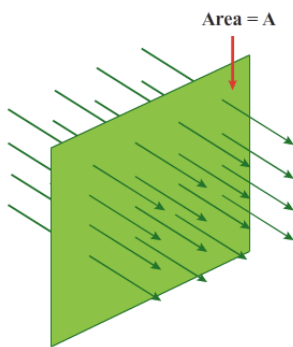
Fig. 21. Se ilustra el flujo eléctrico a través de una superficie de área A.
