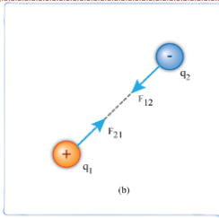
Fig. 7. Se ilustra la fuerza que se ejerce sobre una carga negativa por otra carga del mismo signo.
