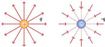
Fig. 16. Líneas de campo eléctrico de una carga positiva y de una carga negativa.
