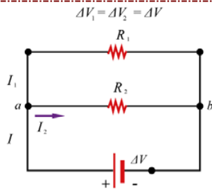
Fig. 42. Resistencias en paralelo y el sentido de la corriente.
