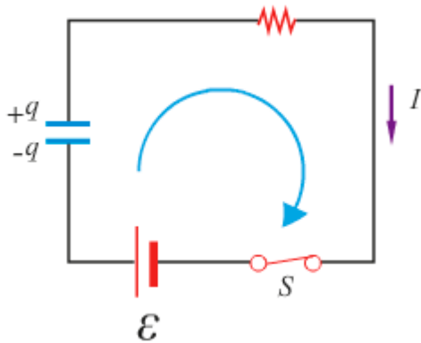
Fig. 47. Análisis del circuito usando la regla de las mallas de Kirchhoff.
