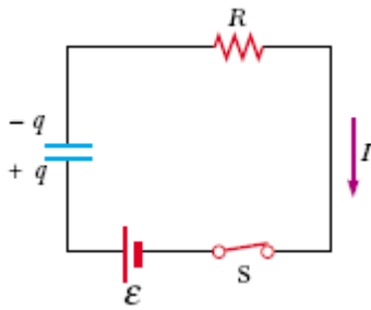
Fig. 46. Circuito que muestra la carga del capacitor.
