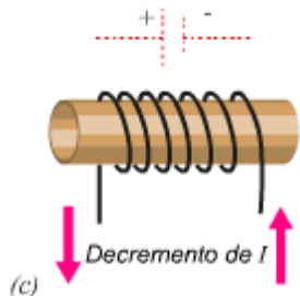
Fig. 53. La FEM autinducida también es contraria al cambio si la corriente disminuye.
