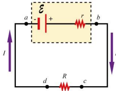
Fig. 37. Se muestra la resistencia interna de la batería.
