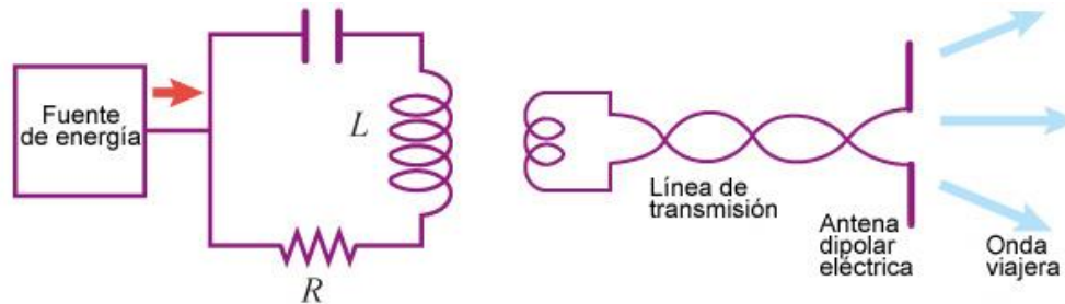
Fig. 35. Circuito que permite generar ondas electromagnéticas viajeras.
