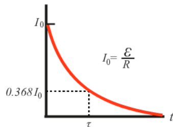
Fig. 49. Variación de la corriente durante la carga del condensador.
