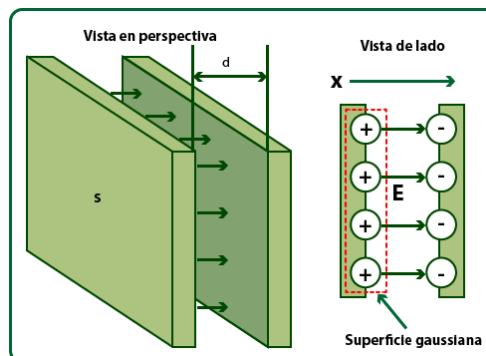
Fig. 44. Capacitor de placas paralelas.
