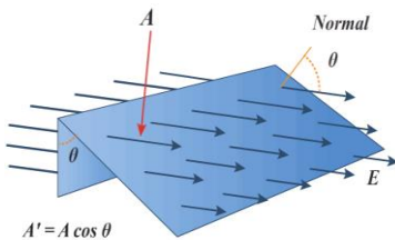
Fig. 22. Flujo eléctrico a través de una superficie de área A no perpendicular al flujo.
