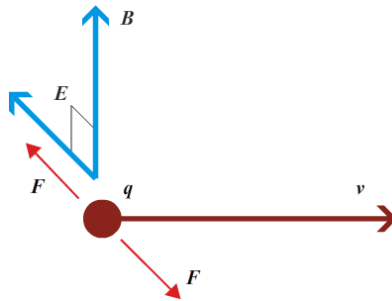
Fig.27 En un campo eléctrico y magnético mutuamente perpendiculares una partícula cargada puede moverse a velocidad constante \vec{v} con magnitud igual a v = \frac{E}{B} , y dirección perpendicular a ambos campos.
