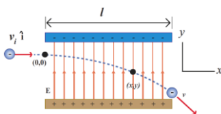
Fig. 17. Una partícula cargada moviéndose en un campo eléctrico uniforme.
