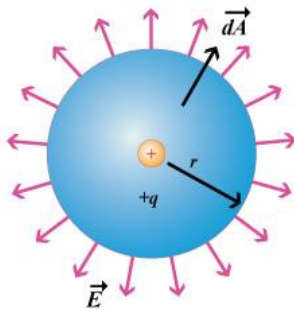
Fig. 24. Superficie Gaussiana esférica alrededor de una carga puntual positiva. El flujo se dirige hacia afuera de la superficie.
