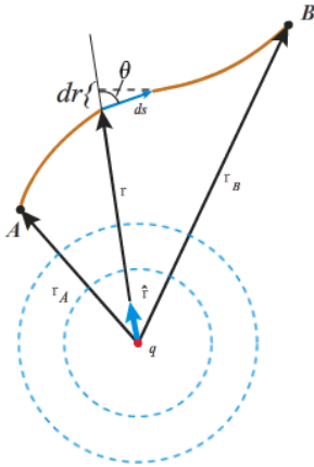
Fig. 18. El potencial eléctrico entre los puntos A y B depende sólo de la distancia radial r_A y r_B a la carga q .
