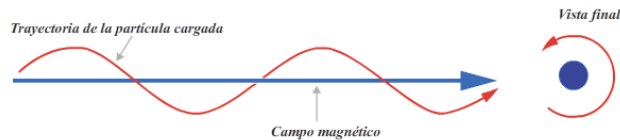
Fig.29. Movimiento en espiral de una partícula cargada en la dirección del campo magnético. El movimiento se compone de un movimiento circular alrededor del vector del campo más un movimiento de traslación a lo largo del campo.
