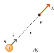
Fig. 11. Campo eléctrico en el punto p .
