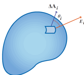
Fig. 23. Flujo eléctrico a través de un elemento de área infinitesimal.
