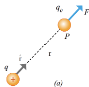
Fig. 10. Partícula cargada de prueba a una distancia r de la carga q .
