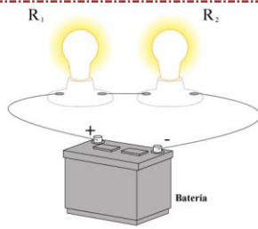
Fig. 38. Circuito con resistencias en serie con una batería.
